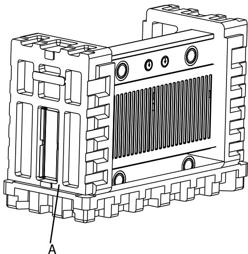
A. Amortiguador de ventilación rectangular de 3¼" x 10" (8,3 x 25,4 cm)
