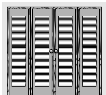
Portes à persiennes pliantes à deux vantaux avec ventilation de 120 po 2
