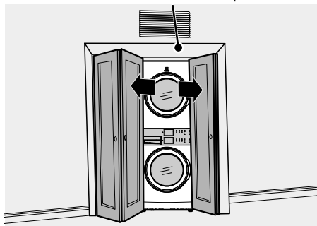
Les portes solides à deux rabats sans ventilation nécessitent une ouverture de porte pour 120 po 2 de ventilation murale
