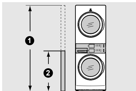
Les portes solides à deux rabats sans ventilation nécessitent une ouverture de porte pour 120 po 2 de ventilation murale
