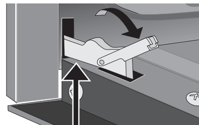
Figure 36: Déverrouillage de la charnière de porte
