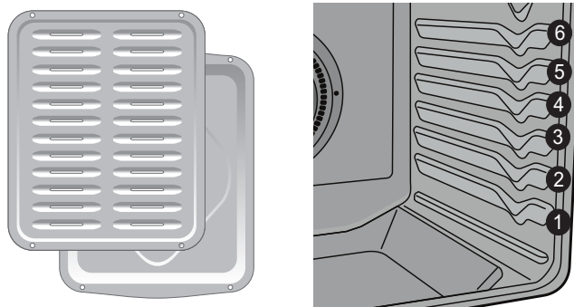
Figure 10 : Lèchefrite avec grille (G) et positions de la grille (D)
