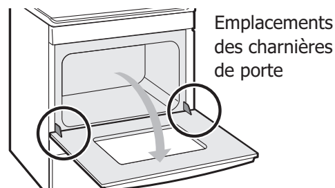
Figure 42 : Emplacement des charnières de porte
