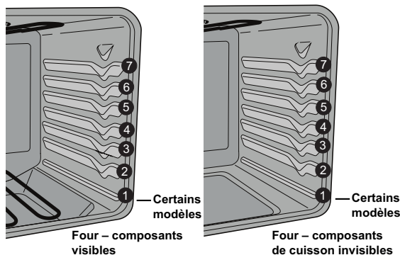
Figure 15 : Emplacement des grilles pour les fours à éléments de cuisson visibles ou dissimulés.
