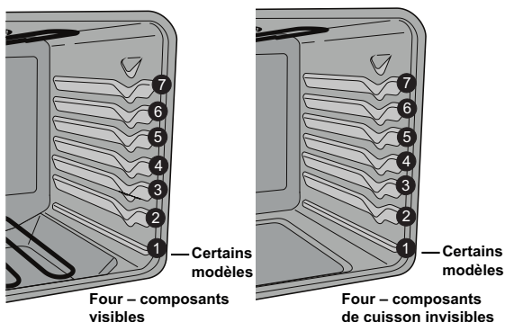
Figure 17 : Emplacement des grilles
