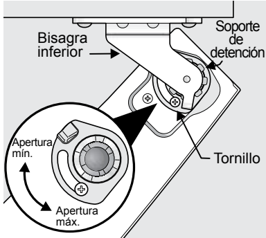
Tope de puerta ajustable
