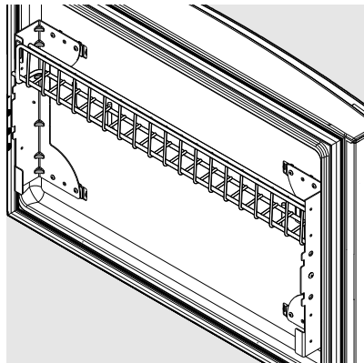
*alambre estante (dentro del cajón del congelador)
