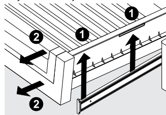
Cómo quitar el cajón
