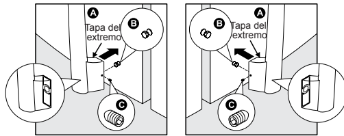
Montaje de las manijas del refrigerador
