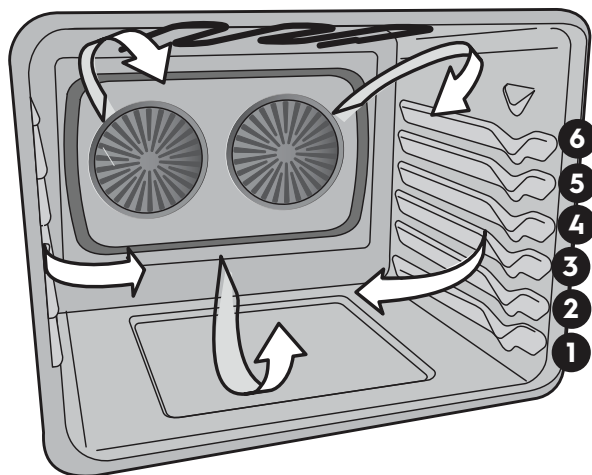
Figure 5 : Rôtissage à convection sur les grilles du four inférieur
