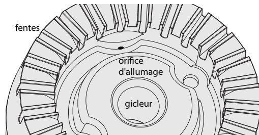
Figure 25 : Têtes de brûleurs à gaz
