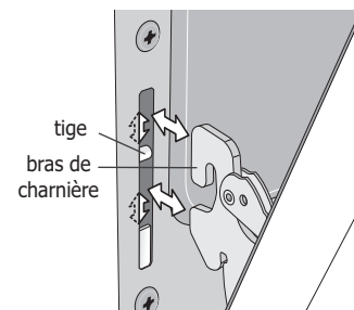
Figure 24 : Remise en place et emplacement des bras de charnière et des tiges
