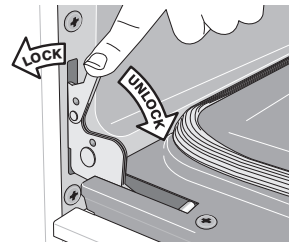
Figure 22 : Verrous de charnière de porte
