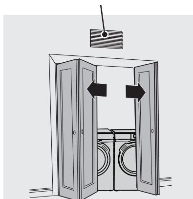
Portes pliantes pleines sans ventilation
