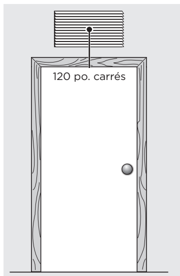
Porte pleine avec ventilation murale
