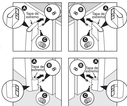
Instalación de las manijas del refrigerador
