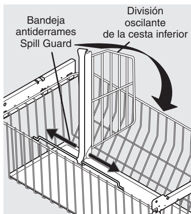
División oscilante de la cesta inferior (algunos modelos)
