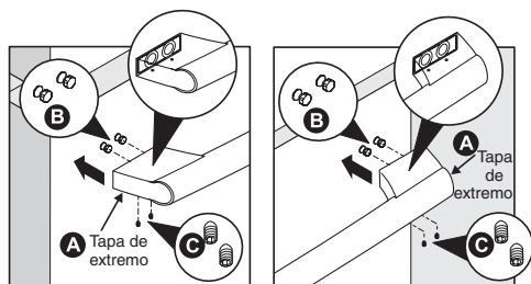
Instalación de la manija del congelador
