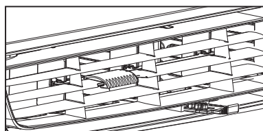
Figura 3 (VENTILACIÓN ABIERTA)
