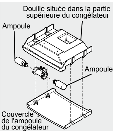
Lumière du congélateur
