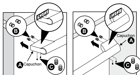
Assembler la poignée du congélateur
