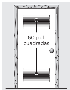
Puerta de ventilación dividida igualmente dividida de 120 pul. cuadradas
