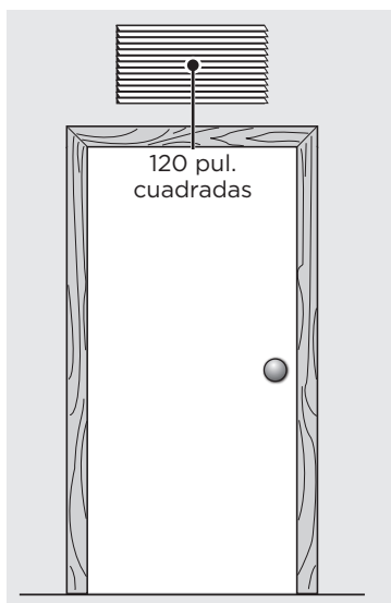
Puerta sólida con ventilación de pared
