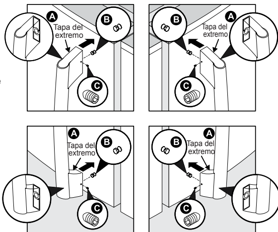
Montaje de las manijas del refrigerador
