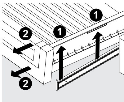
Cómo quitar el cajón
