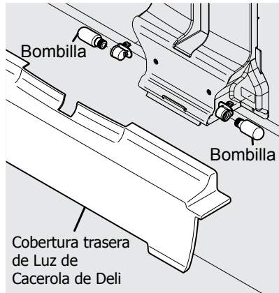
Luz en la pared trasera
