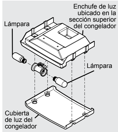
Luz del congelador
