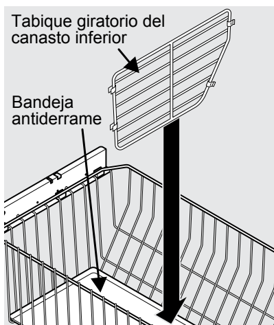
Tabique del canasto inferior y bandeja antiderrame
