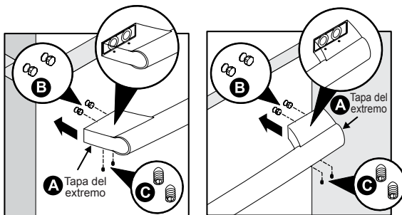
Montaje de la manija del congelador
