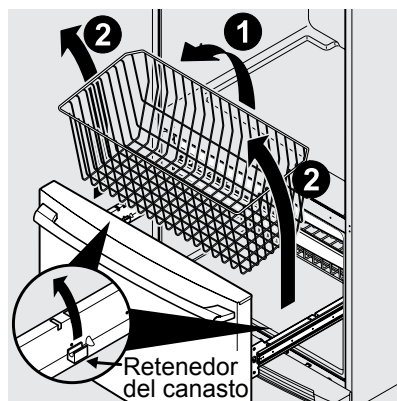
Para quitar el canasto inferior
