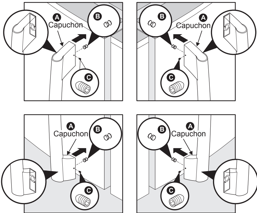
Assembler les poignées du réfrigérateur
