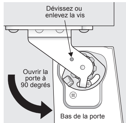
Desserrez/retirez la vis (s'il y a lieu)
