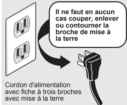
Prise murale avec mise à la terre
