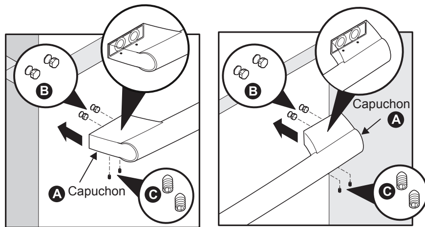
Assembler la poignée du congélateur
